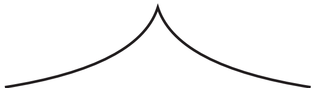
Tractrix
