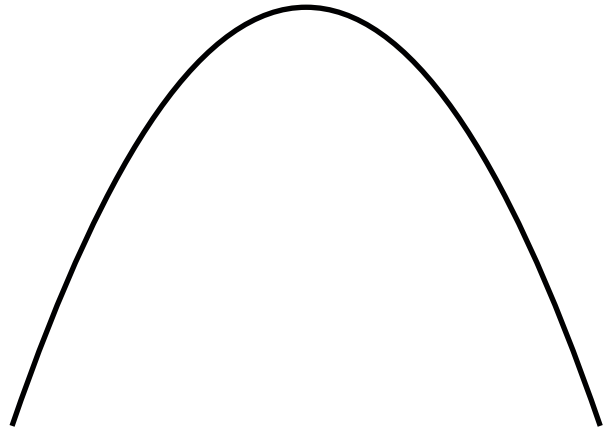
Parabola
